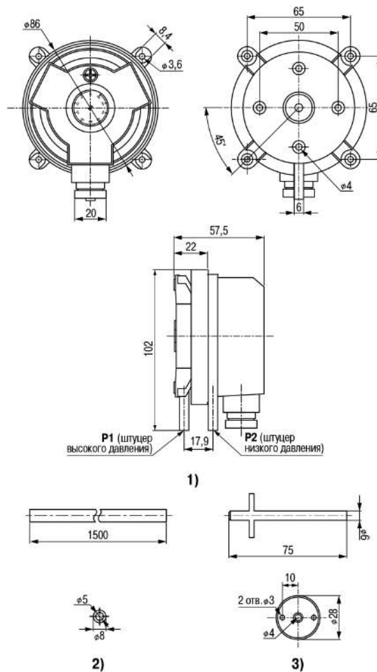
Рисунок 4.1 – Габаритные и присоединительные размеры прибора (1), импульсной трубки (2) и монтажных адаптеров (3)
